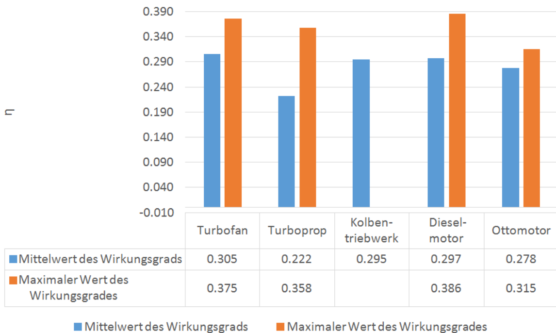
Figure 1: Mittelwert und Maximalwert des Wirkungsgrads verschiedener Flugzeugtriebwerke
