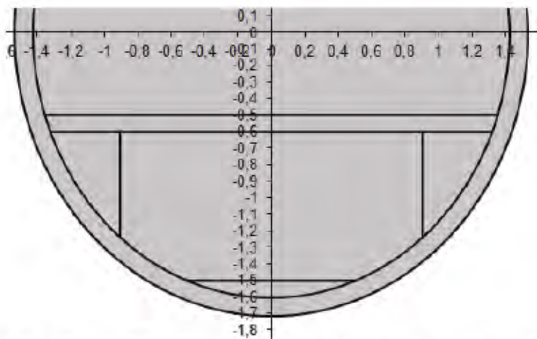
Bild 4.23 Mit PreSTo-Cabin erzeugter Frachraumquerschnitt der ARxxx-4-Familie
