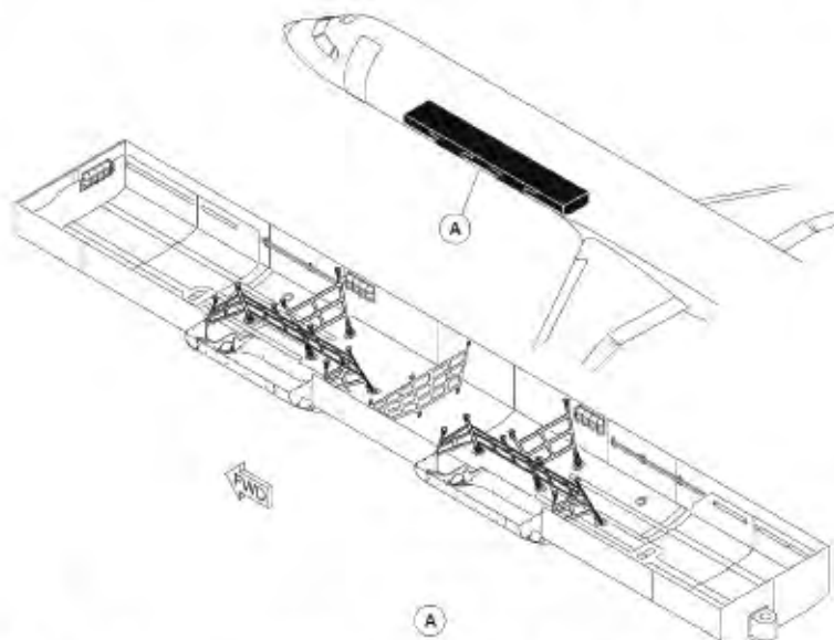
Bild 4.11 Unbegehbbarer Frachtraum der Bombardier CRJ900 (Bombardier 2005)
