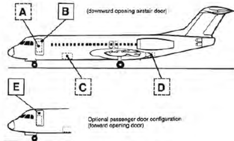
Bild 3.1 Seitenansicht der F70 (AHM 2012)
