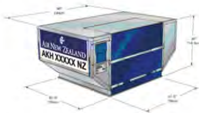
Bild 2.2 LD3-45W Container (First Global 2012)
